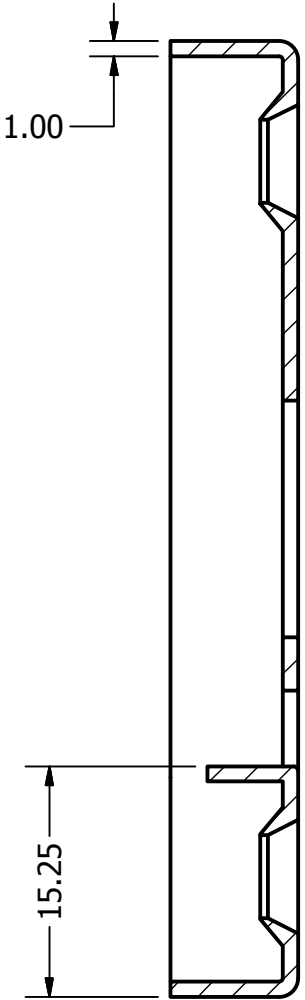
SECTION A-A SCALE 2 : 1
